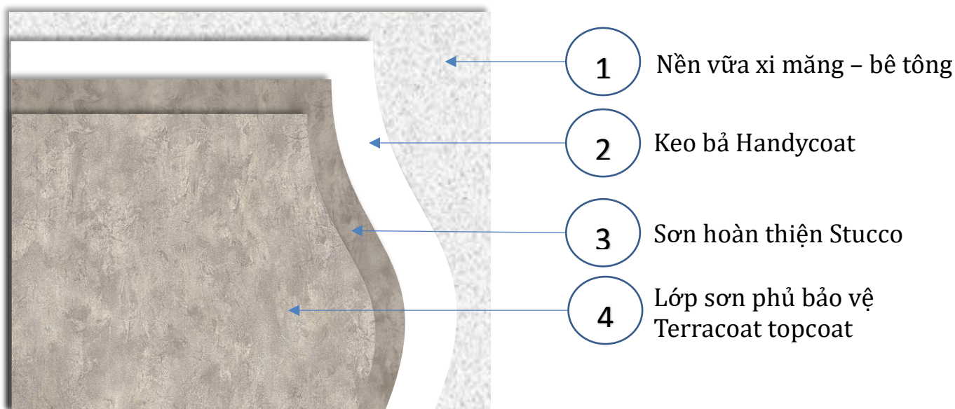
Hình 2. Cấu tạo hệ thống sơn hiệu ứng bê tông
